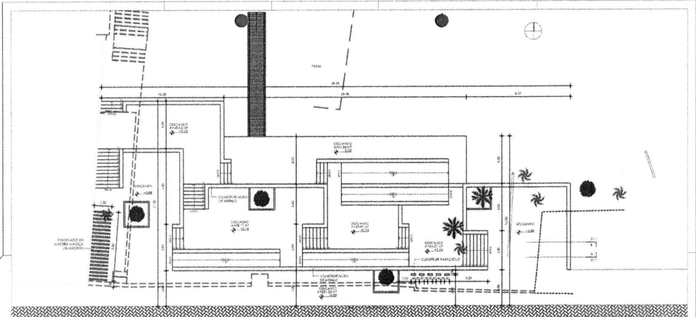
01 PLANTA DEMOLIR/CONSTRUIR
