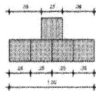
04 DET. ENCONTRO PISO PODOTÁTIL escala 1:50
