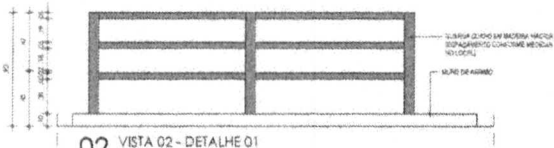
02 VISTA 02 - DETALHE 01 escala 1:20
