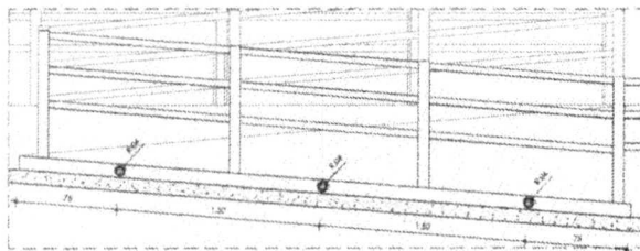
06 CORTE AA - DETALHE 04 escala 1:20
