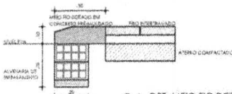
06 DET. MEIO FIO DEIXADO escala 1:10
